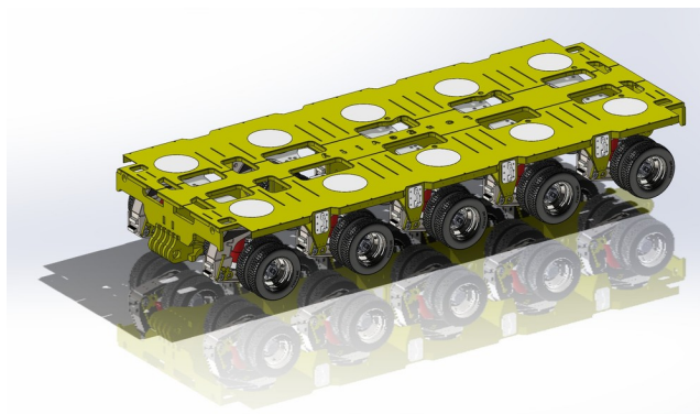
5-osovinski modul
